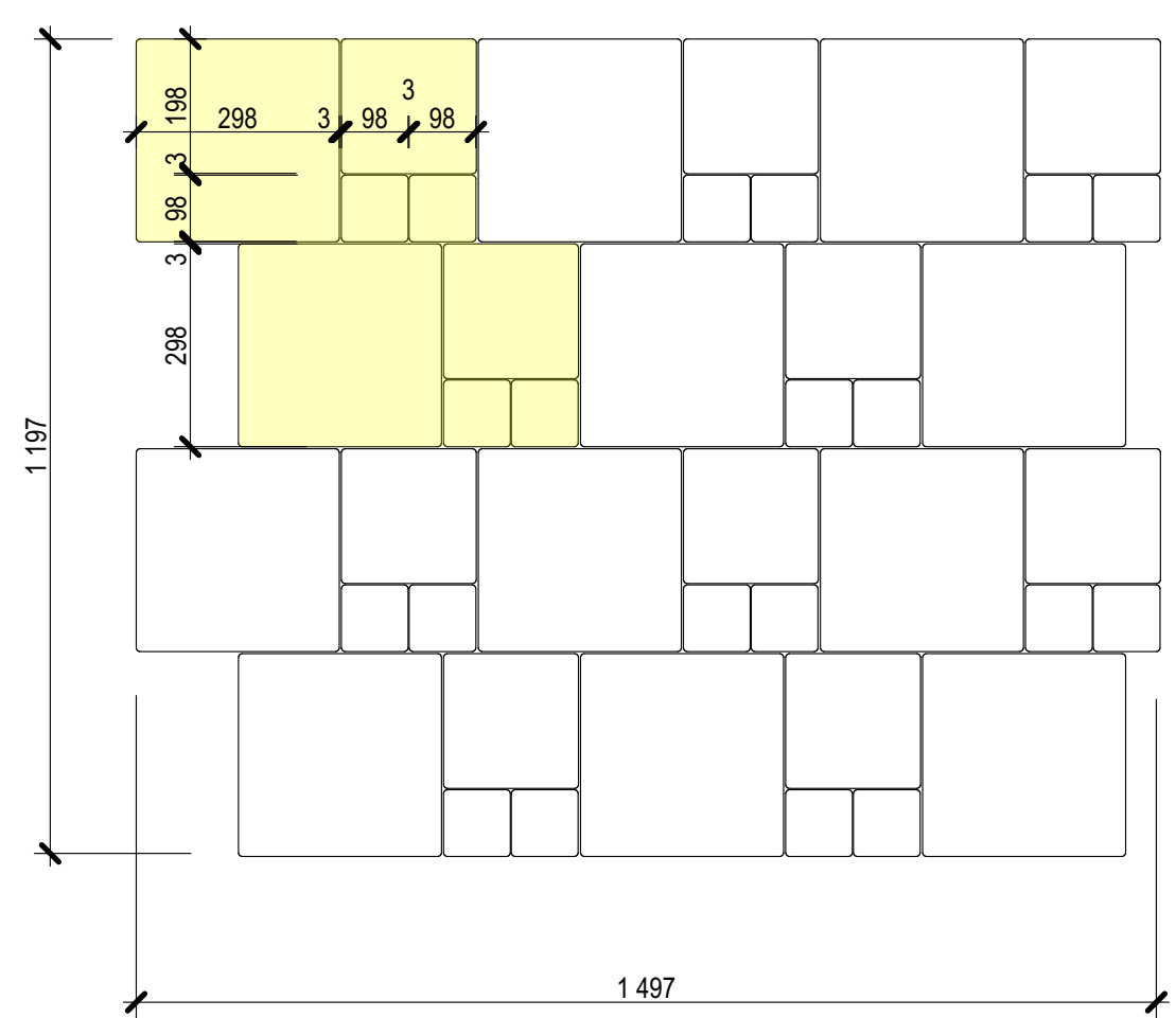
КВАДРАТ 100х100+КВАДРАТ 300Х300+КВАДРАТ 200Х200
