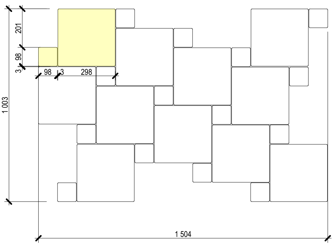
КВАДРАТ 100х100+КВАДРАТ 300Х300
