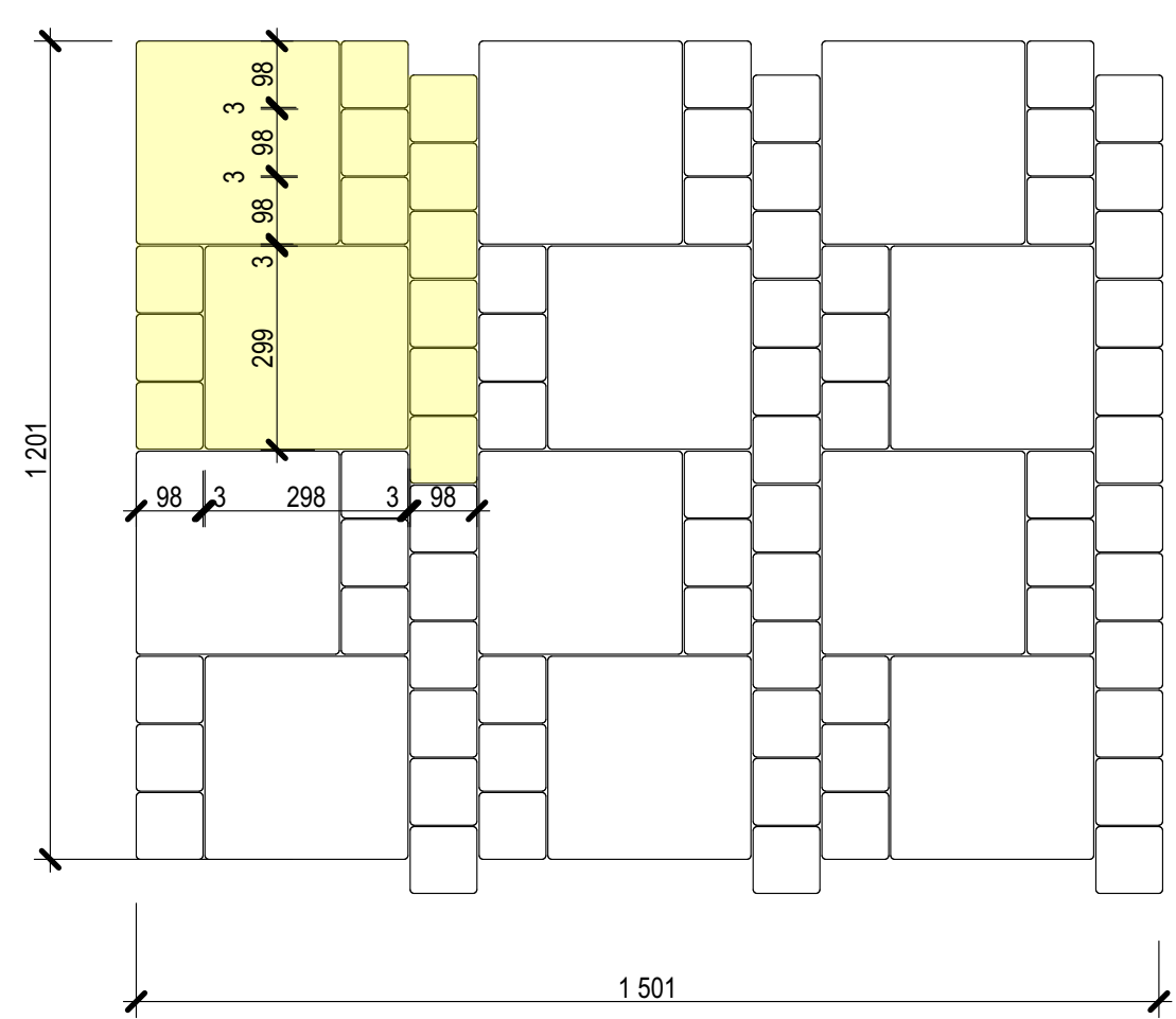
КВАДРАТ 100х100+КВАДРАТ 300Х300
