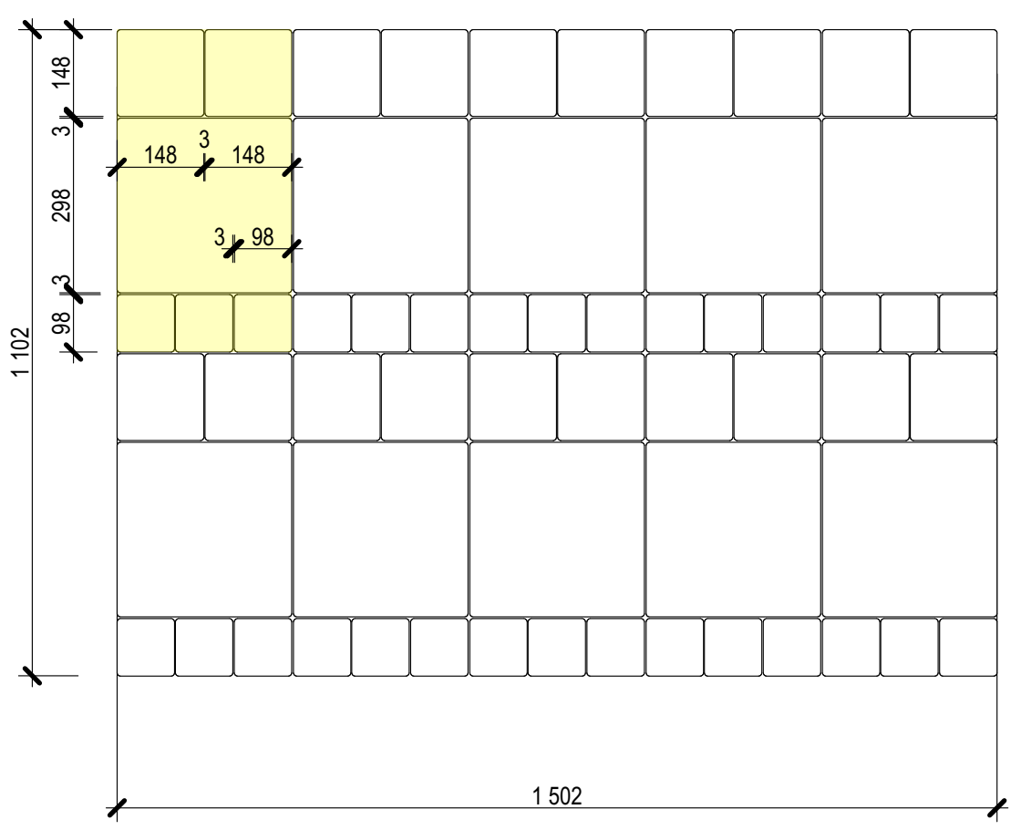
КВАДРАТ 100х100+КВАДРАТ 300Х300+КВАДРАТ 150Х150
